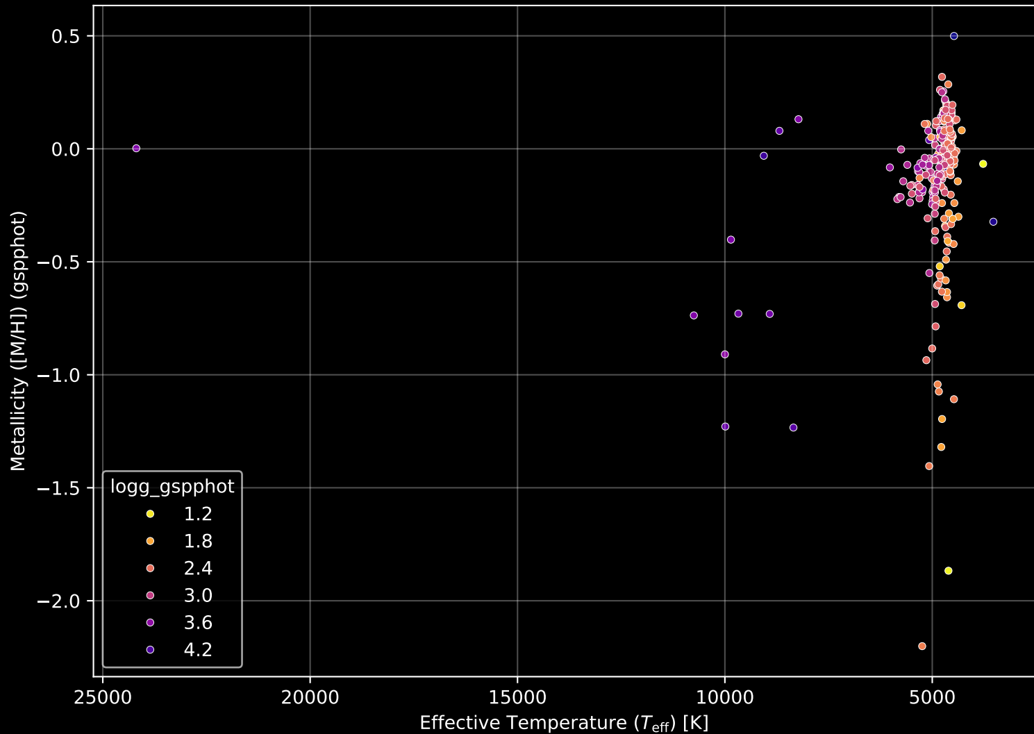
APOGEE DR17 Field: [296+06] Stellar Population Parameters (n= 261)
